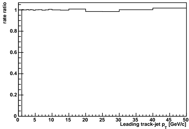
Nal_Vs_LdgJetPt_UE
