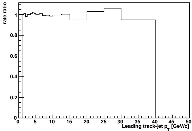
Nla_Vs_LdgJetPt_UE
