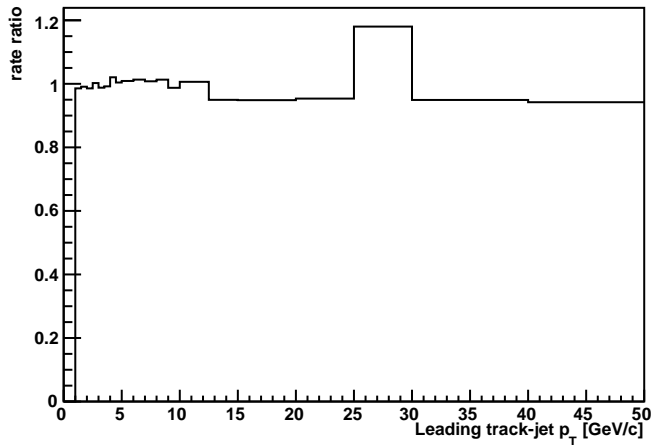
Nal_Vs_LdgJetPt_UE
