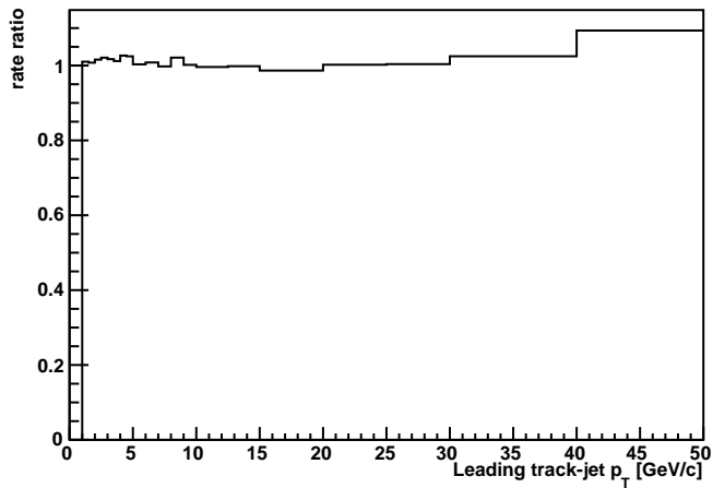
Nal_Vs_LdgJetPt_UE_corr
