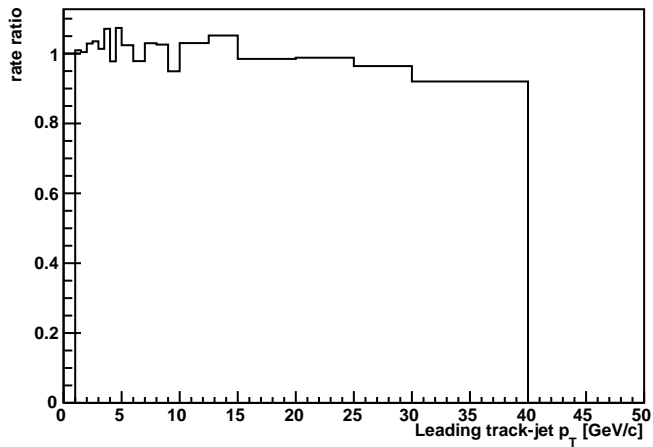
Nla_Vs_LdgJetPt_UE_corr
